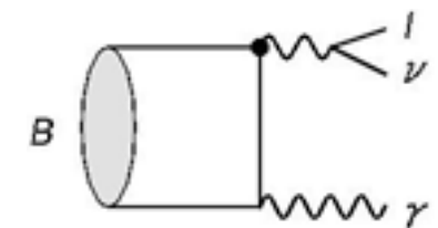
図2: B中間子の輻射崩壊
